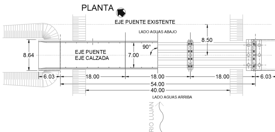
Figura 7: Estructura vista en planta
