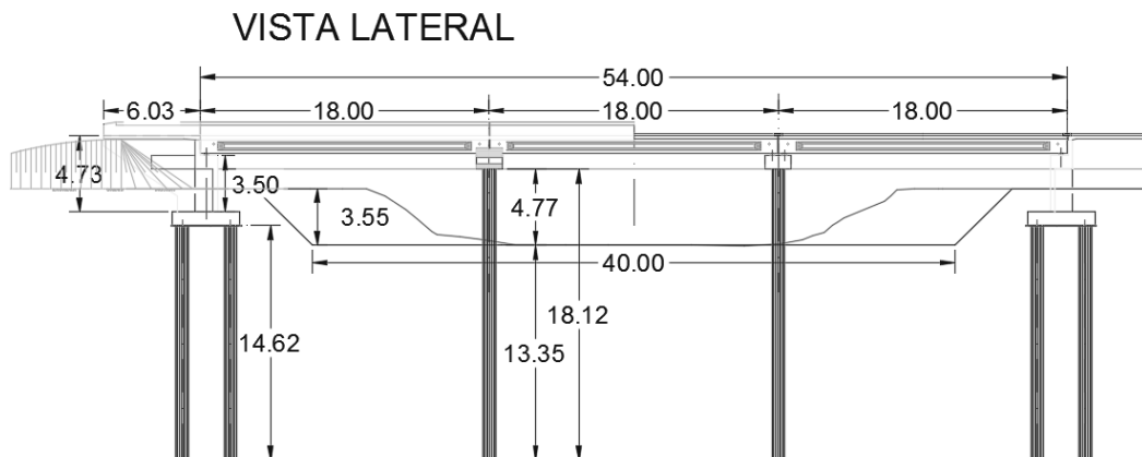
Figura 6: Estructura. Vista lateral
