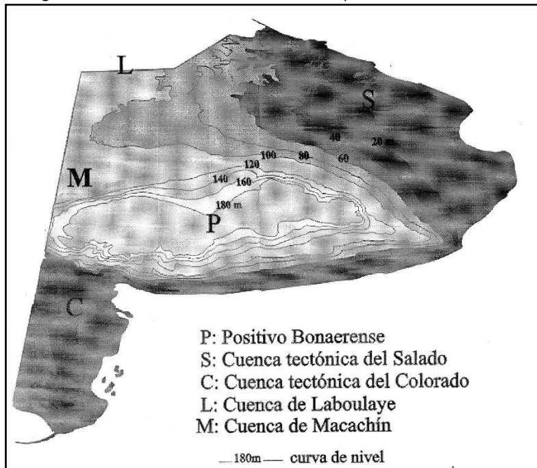
Figura 15: Elementos morfoestructurales de la provincia de Buenos Aires.
