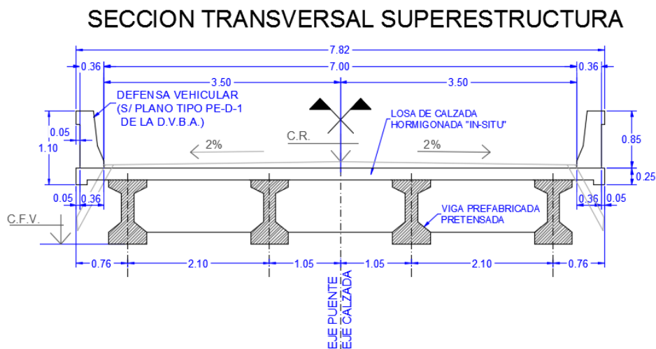
Figura 5: Sección transversal de la superestructura
