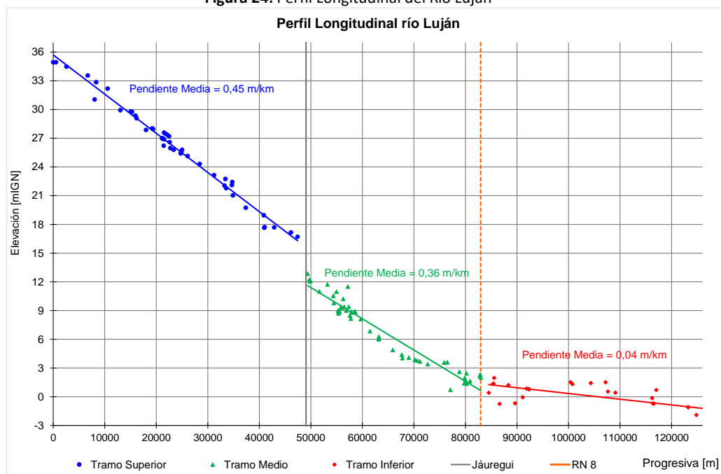
Figura 24: Perfil Longitudinal del Río Luján
