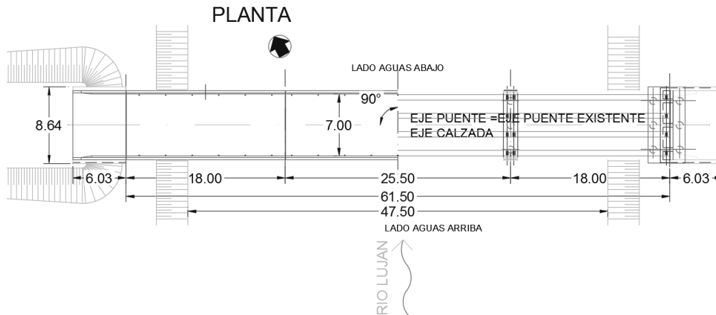
Figura 6: Estructura vista en planta
