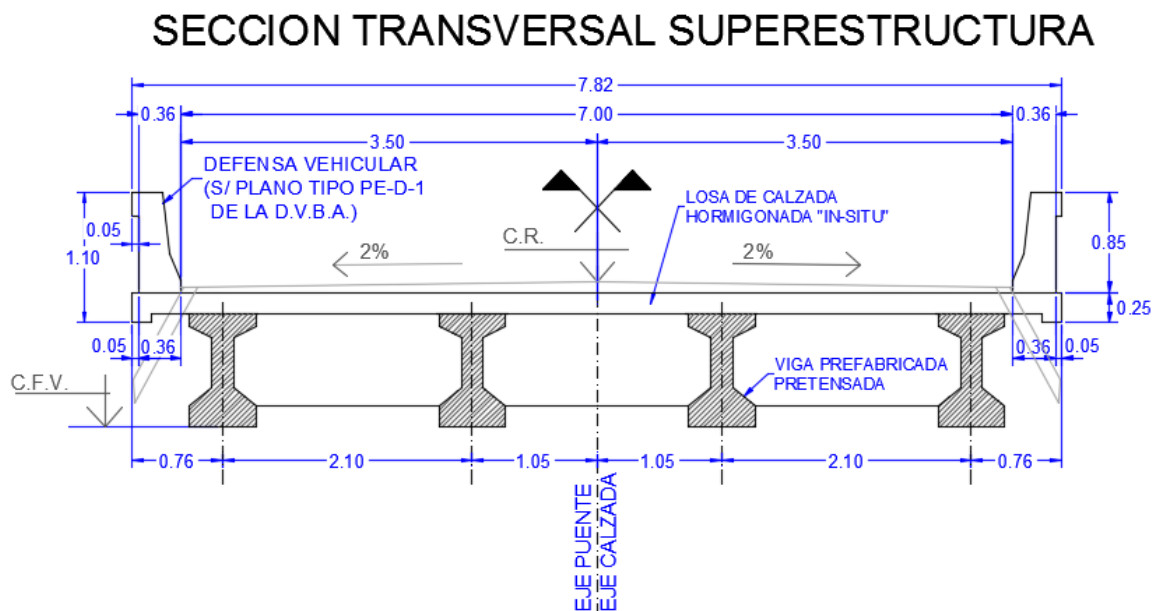
Figura 4: Sección transversal de la superestructura
