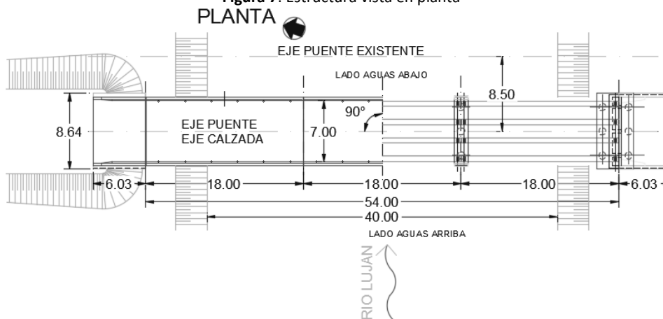
Figura 7: Estructura vista en planta
