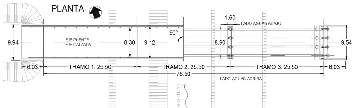
Figura 6: Estructura vista en planta
