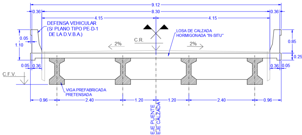
Figura 4: Esquema de ubicación del nuevo puente SECCION TRANSVERSAL SUPERESTRUCTURA
