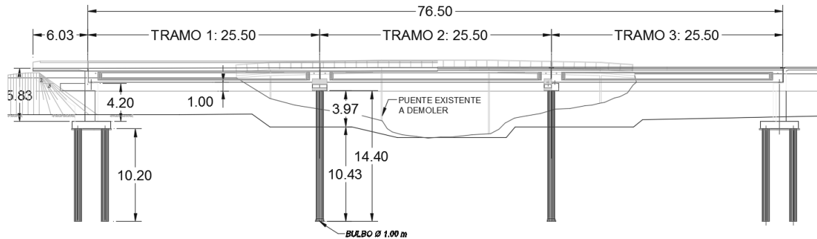
Figura 5: Estructura. Vista lateral VISTA LATERAL
